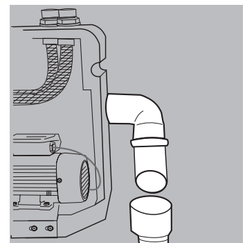
Anschlussbeispiel
