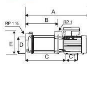
Abmessungen [mm]
