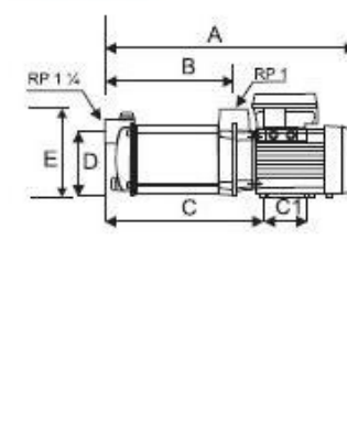
Abmessungen [mm]
